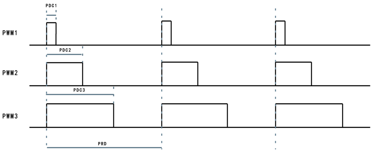
3 路共周期 PWM 时序说明
