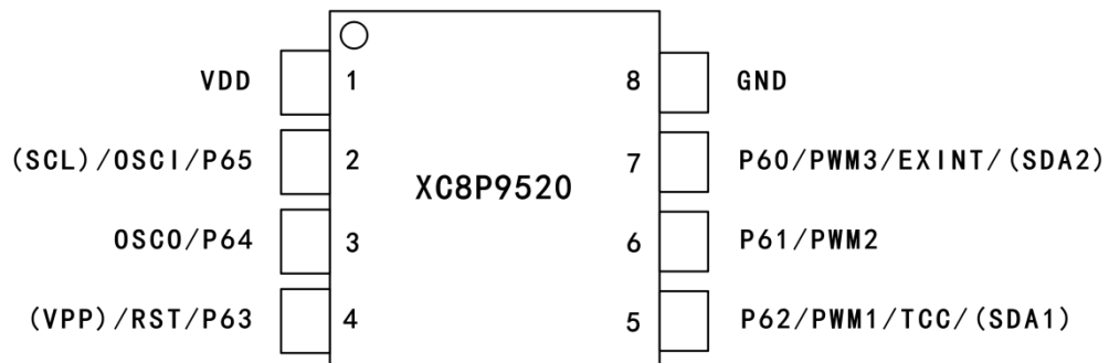
XC8P9520-8PIN 脚位图
