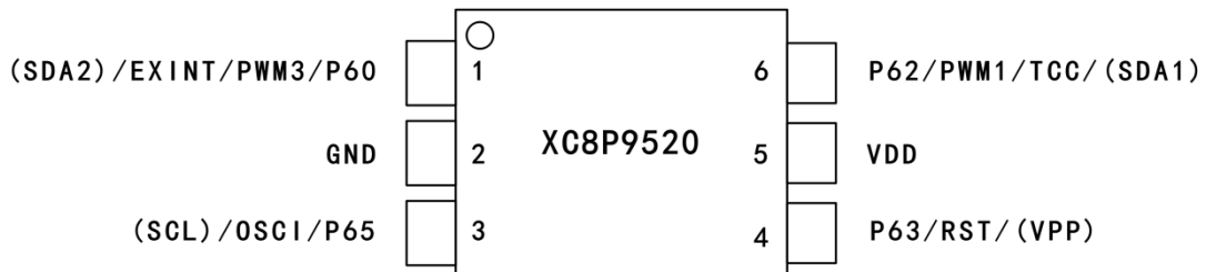
XC8P9520-6PIN 脚位图
