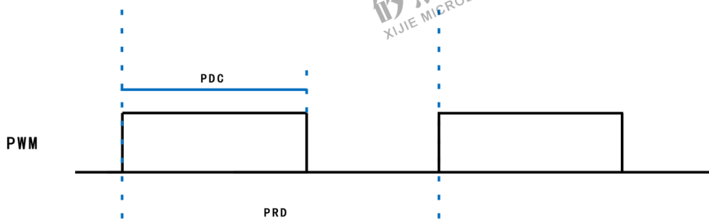
3 路共周期 PWM 时序说明
