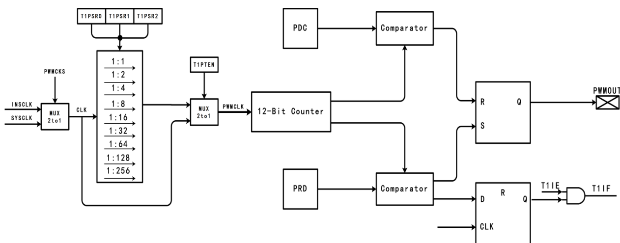
PWM 工作结构电路
