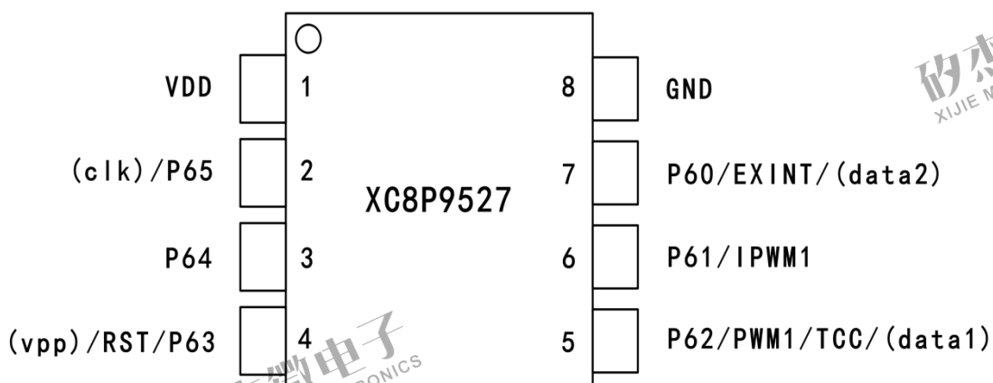
XC8P9527-8PIN 脚位图
