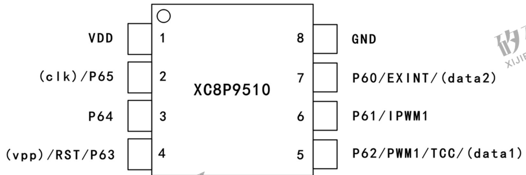
XC8P9510-8PIN 脚位图
