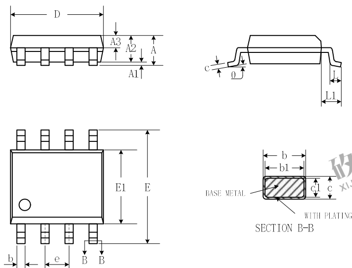
SOP8
