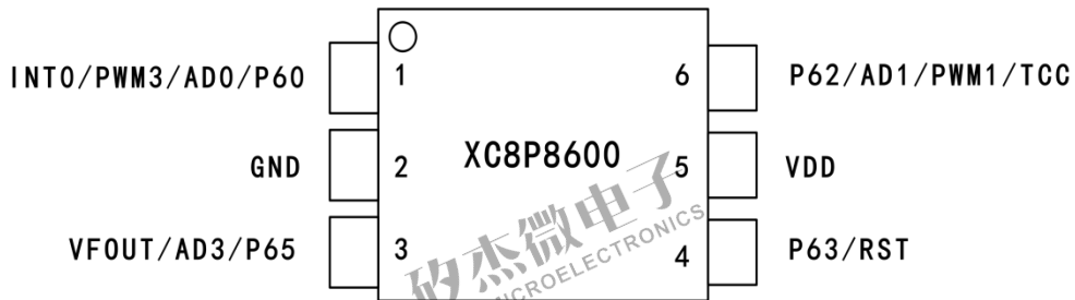
XC8P8600-6PIN 脚位图
