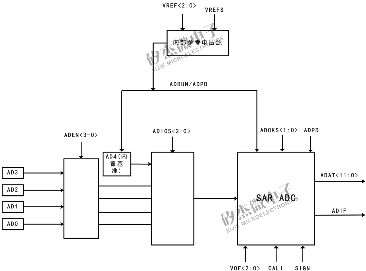
ADC 结构框图
