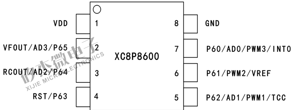
XC8P8600-8PIN 脚位图
