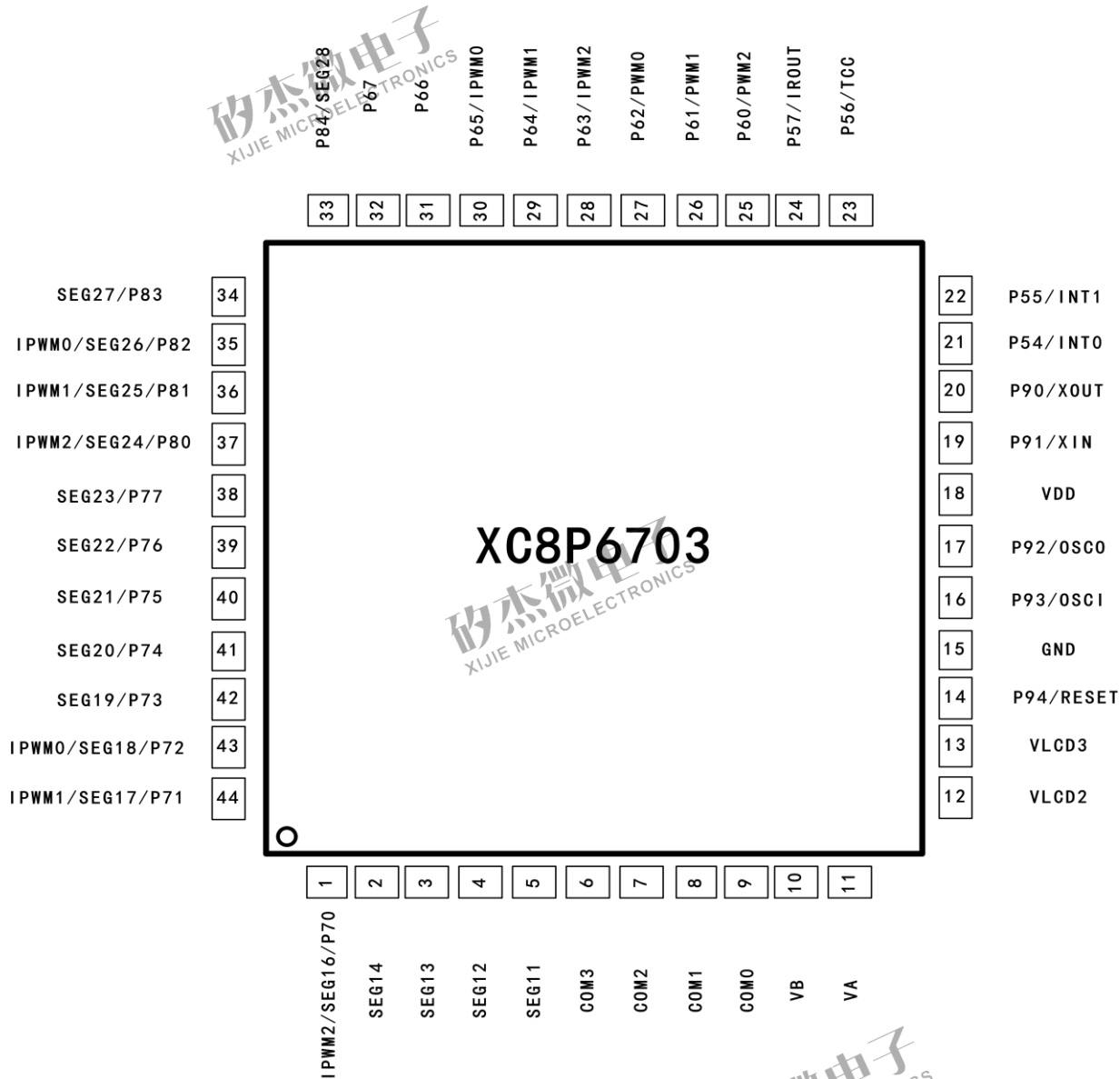
XC8P6703-44PIN 脚位图
