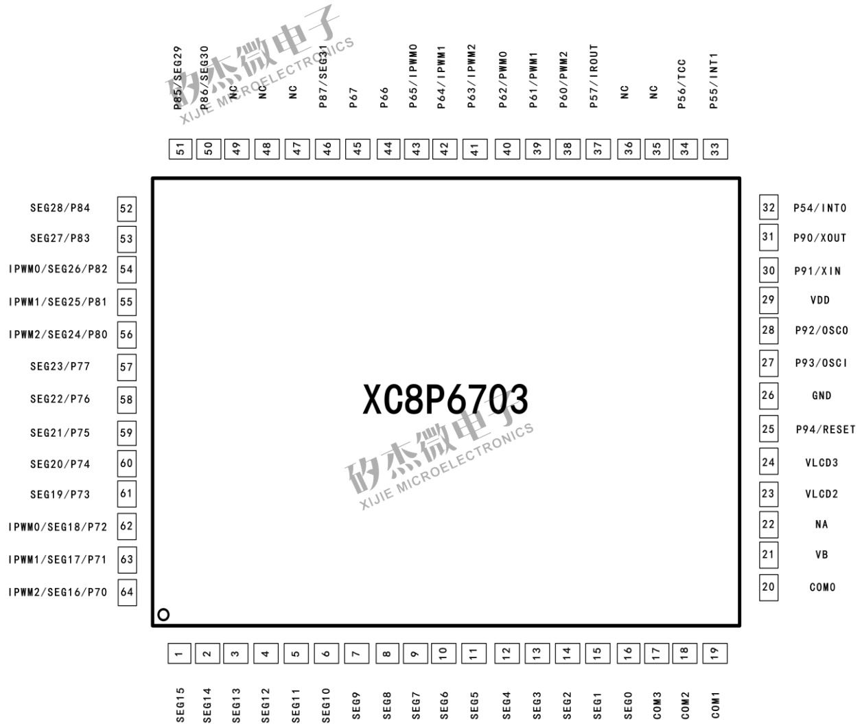
XC8P6703-64PIN 脚位图
