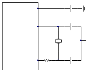
PLL 模式电路
